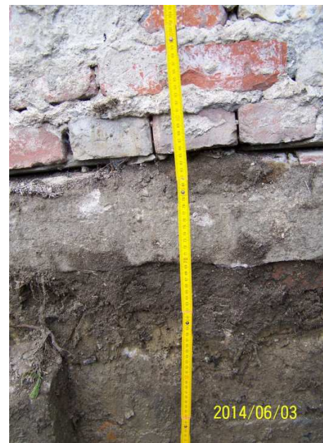
Fot . 12 Ściana południowa – Odkrywka fundamentu, brak izolacji poziomej i pionowej
